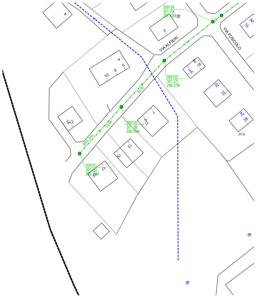
ESTRATTO MAPPE FOGNARIE SMAT
