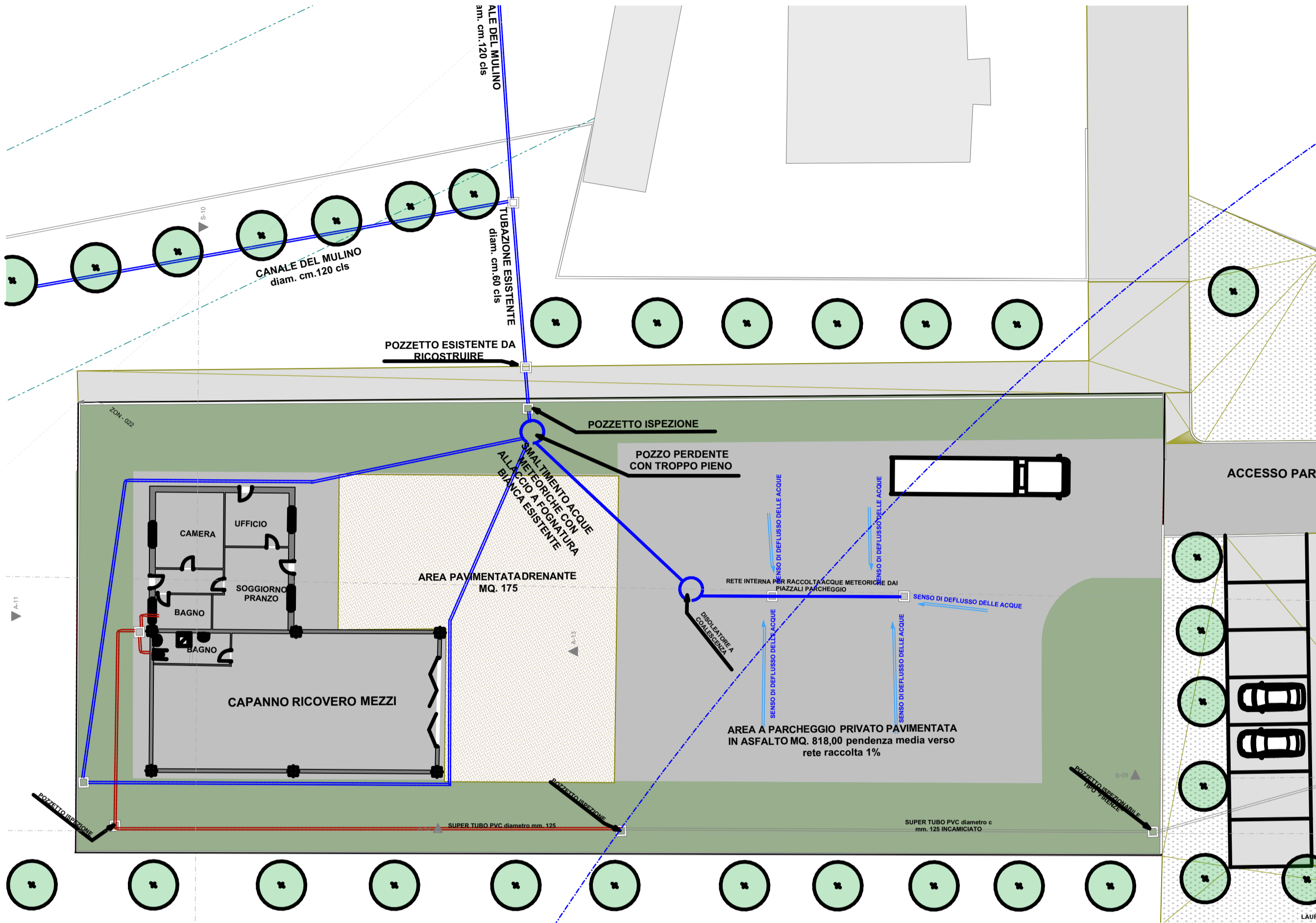
PLANIMETRIA scala 1:250
