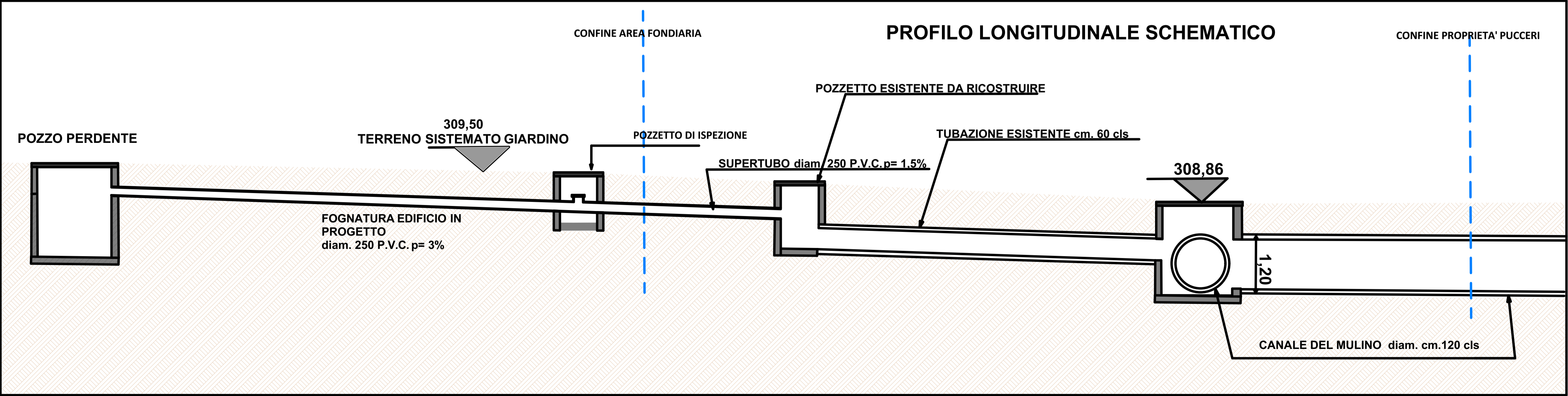
SCHEMA ALLACCIO FOGNATURA BIANCA CANALE DEI MULINI
